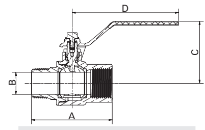
Mit Flachhebel aus Edelstahl AISI 304 With AISI 304 stainless steel flat lever
